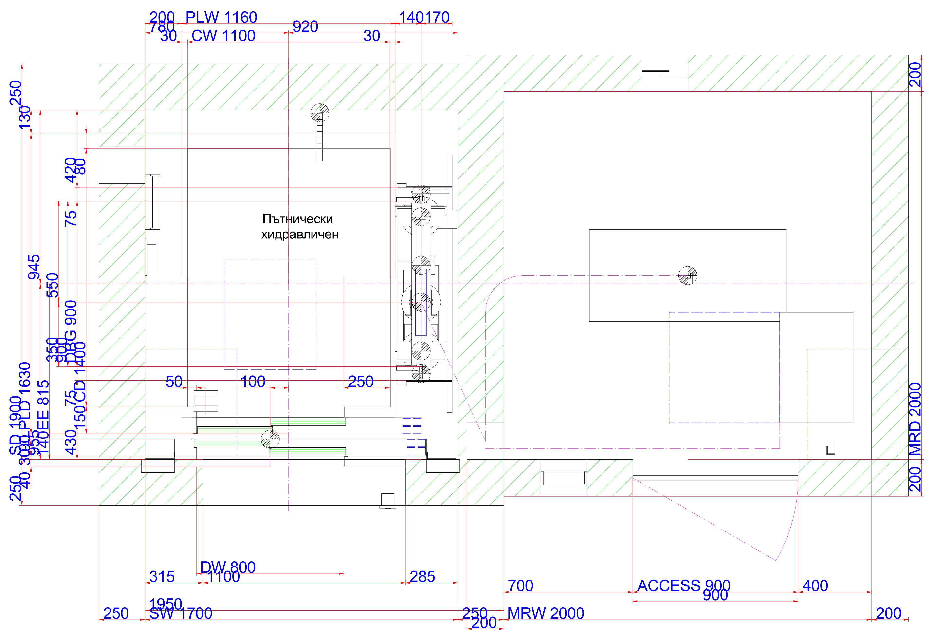
Машинно помещение Мащаб: 1:10
