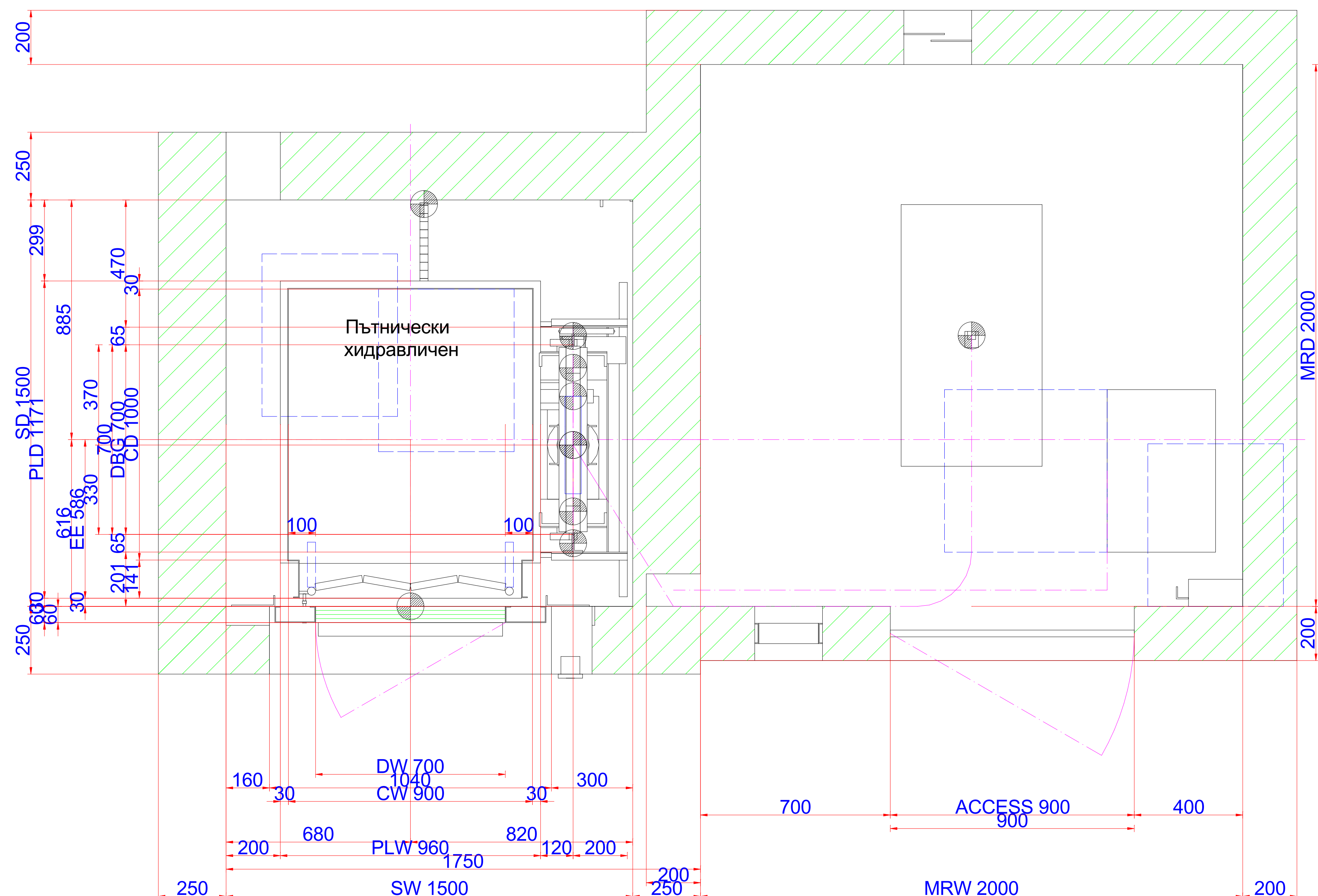
Хоризонтален разрез
