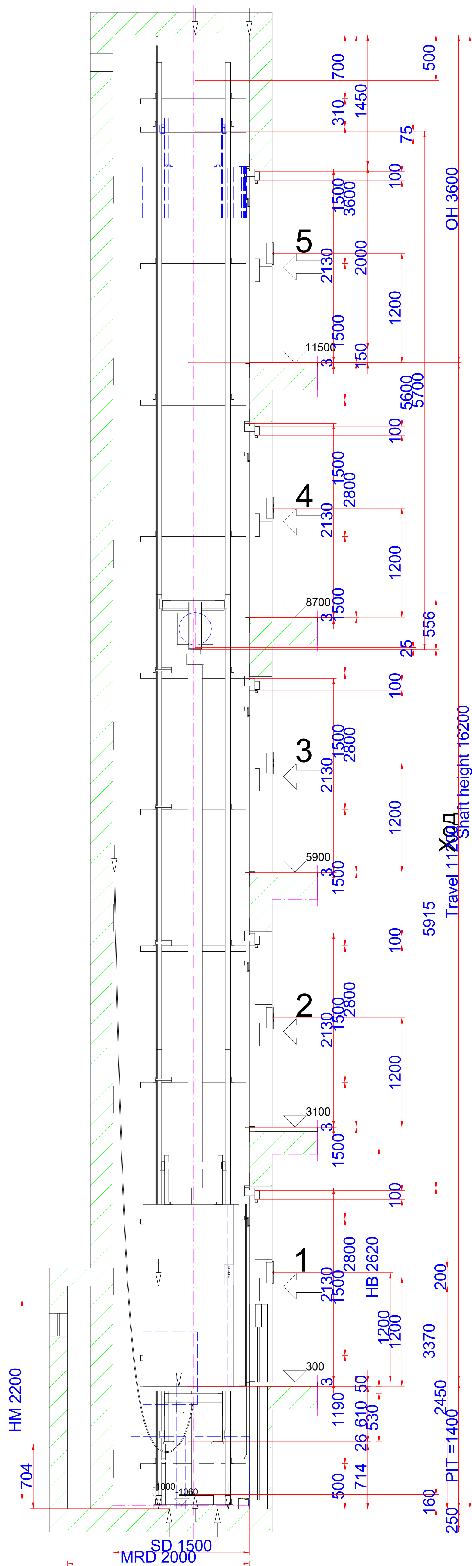
Вертикален разрез Мащаб: 1:25
